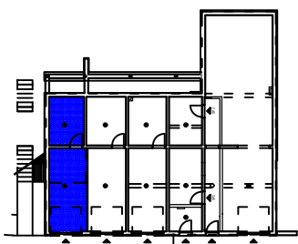
TLOCRT PODRUMA
