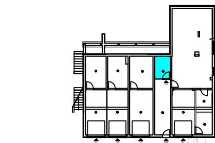
TLOCRT SUTERENA
