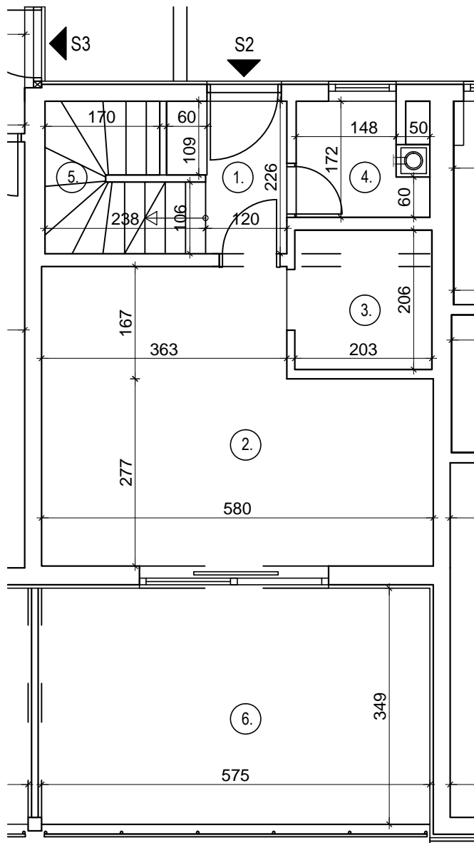
TLOCRT STANA (prizemlje)
