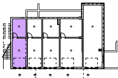
TLOCRT SUTERENA
