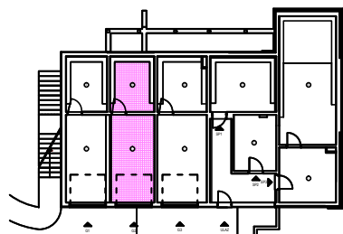
TLOCRT PODRUMA
