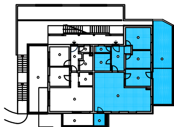
TLOCRT PRIZEMLJA
